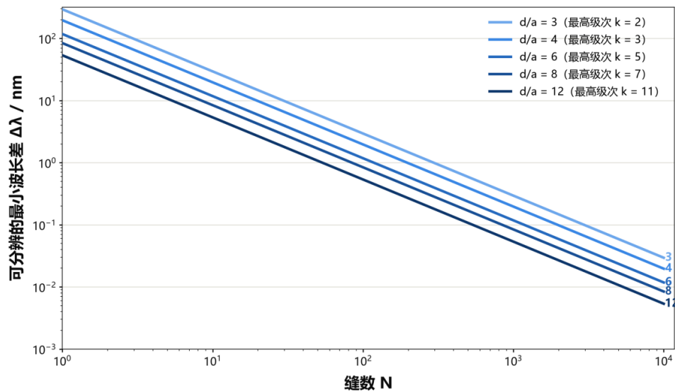
图 3.5: 可分辨的最小波长差随缝数的变化
